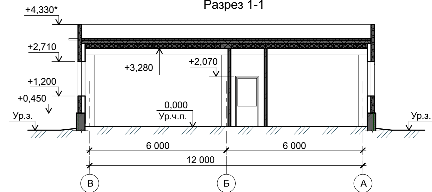
Разрез 1-1
